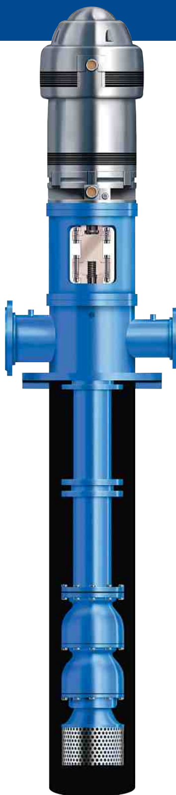
Tipo "T" Entrada de succión ubicada en la cabeza
