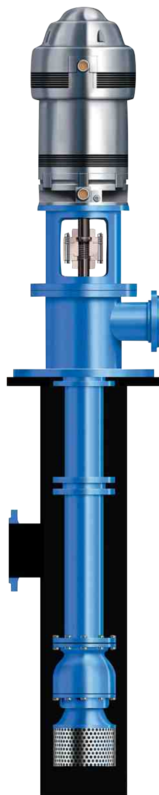
Tipo "L" (Barril) Entrada de succión localizada en la barril
